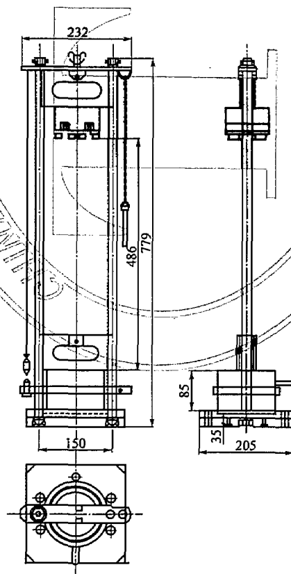
图1 标准集料冲击韧度机
